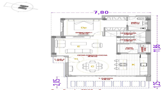
TIPO-05 VIVIENDA Nº: 18 PL/ BAJA. Sup. Const.: 78'37 m2
